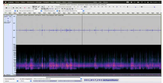
Spectrogramme des clangs de Éliot, toutes les secondes environ
