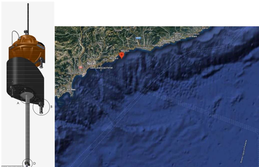
Figure 4.2 : (gauche) Schéma de la Bouée GLAS BOMBYX-2 à 5 hydrophones et son système de ballast (hauteur totale de 3m). (droite) Localisation géographique de BOMBYX-2 face aux rails de trafic maritime (en pointillés).
