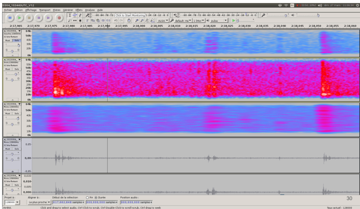
Figure 12.1 : Mesures de l'antenne Stochaedes Rayol le 4 mars 2022, montrant un cachalot détecté vers 15h34, d'IPI environ 2.5 ms. (Haut) En temps, sur les 5 hydrophones. (Bas) En temps-fréquence.
