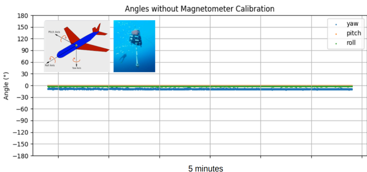
Figure 4.3 : Mesures, par la Motion Process Unit, des trois angles de position de la bouée BOMBYX-2 en juillet 2022. L'assiette est donc très stable.
