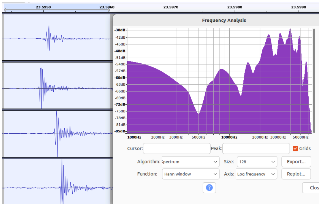
Figure 12.9 : Détection d'un clic d'odontocète, 0,1 ms de long, 3 battements, fréquence centroïde vers 40 kHz mais déjà dans l'antialiasing et perte en dB (signal du 8 août 2021 à 0:54).
