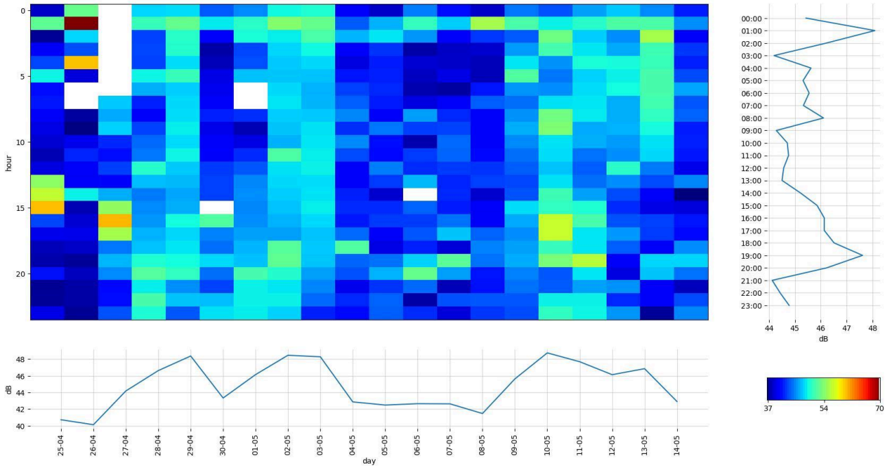
KM3Net_max_dsp_2021_6500-12500_Hz
