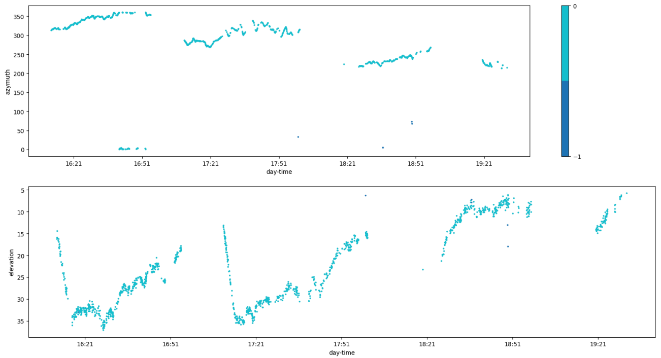
Figure 9.6 : Suivi des mesures d'azimut et d'élévation de l'individu Survivor durant 3 plongées complètes ; la période de descente et de remontée progressive, le 25 septembre 2023.
