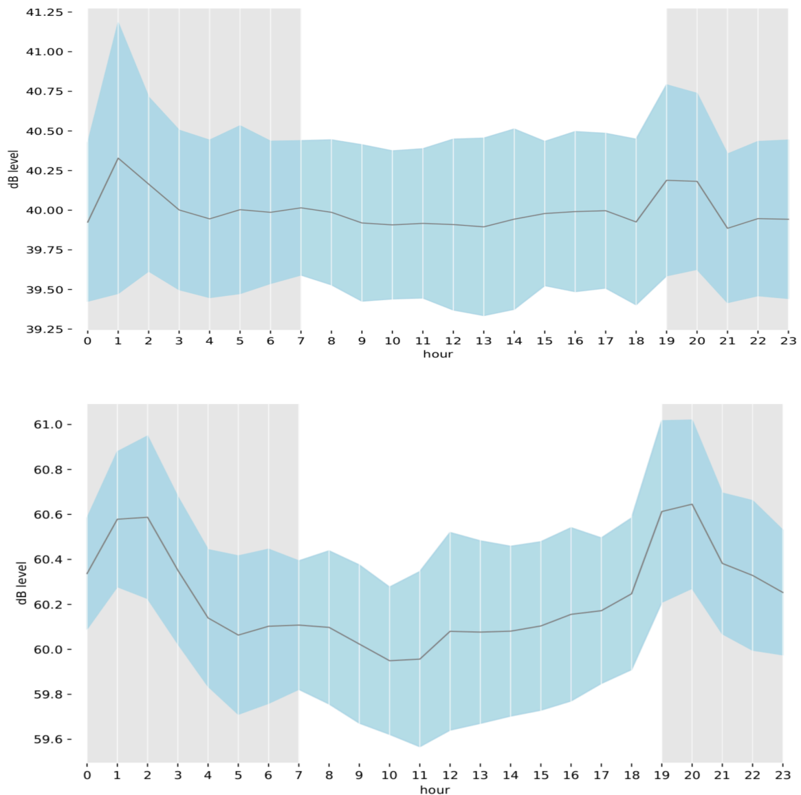
Figure 16.2 : Moyenne du niveau dB dans la plaine abyssale, 20 km au Sud des Iles d'Or, via KM3Env, au fil des heures UTC (=h locale -2), d'une journée moyenne en mai 2020 et mai 2021, nuit (gris) vs jour (clair), écart-type (bleu) sur différentes plage de fréquence. (Haut) bande 10 Hz, 800 Hz, (Bas) bande 6,3 kHz 12,5 kHz. Cela montre la caractéristique d'un trafic maritime polluant un large spectre fréquentiel et à horaires récurrents.
