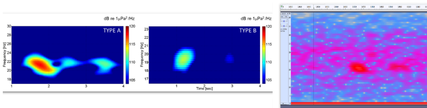
Figure 5.1: Spectrogrammes de trois pulses de rorqual commun de type 18 Hz à 22 Hz.
