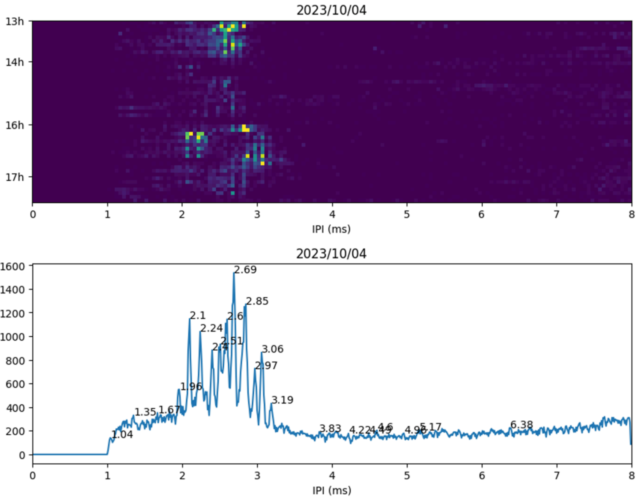
Figure 10.3 : (Haut) Suivi de la piste en IPI (Intervalle inter pulse) entre 13h00 et 17h30, le 4 octobre. (Bas) Histogramme des Intervalles inter pulse de la piste montrant le nombre d'individus et leurs IPI. Ici un groupe de 8 ou 9 individus de tailles petite à moyenne, dont certains sont des immatures (pour les IPI < 2.8 ms).
