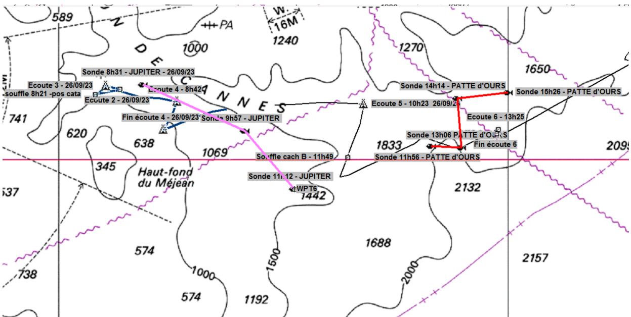
Figure A4.2: (Haut) Suivi réalisé le 26 septembre 2023 pendant la mission WhaleWay-4 (Bas) Zoom sur le suivi de deux individus: Patte d'ours en rouge, et Jupiter en rose.
