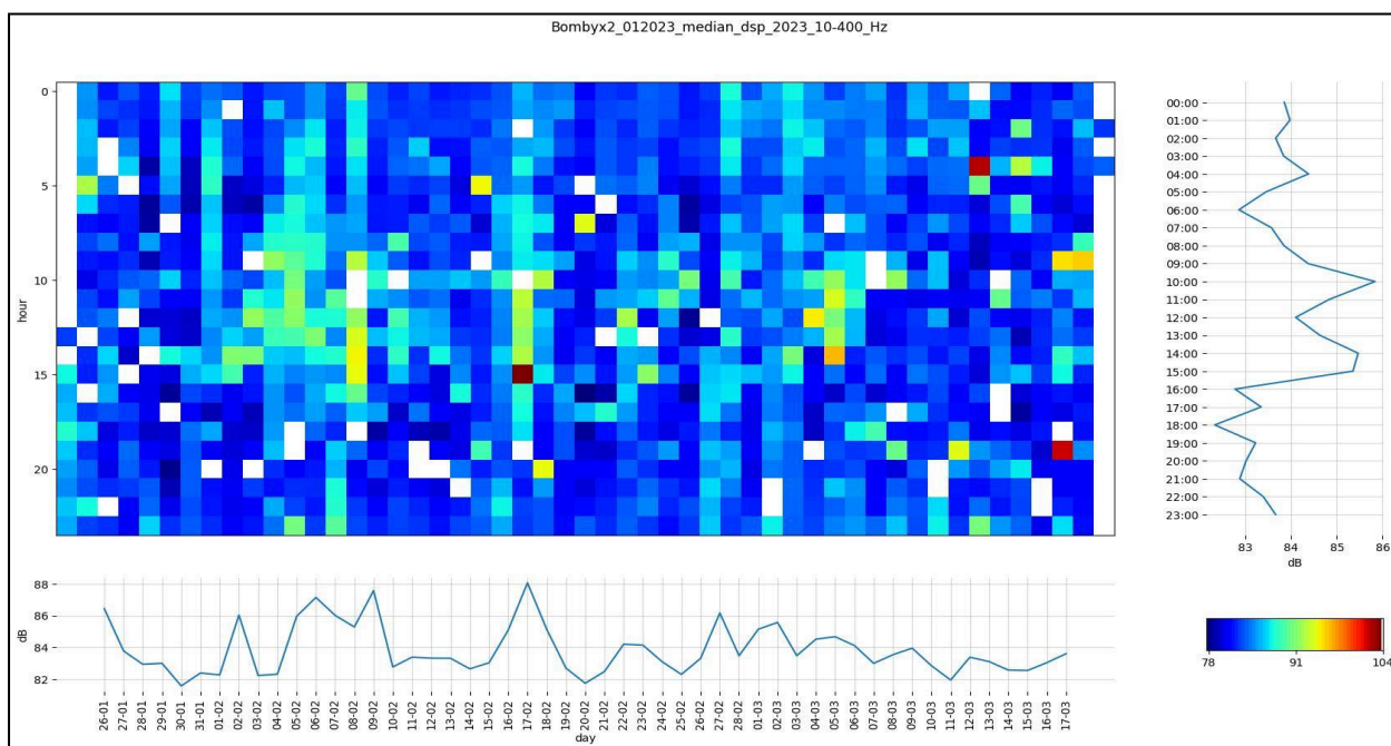
Figure 18.3 : Niveau de bruit médian sur la bande 10 Hz à 800 Hz du début 2023 montrant que l'écoute pour rorqual commun est propice sauf lors d'évènements de ragage de ligne de mouillage ou de galets sur le socle (communication du CIRA).
