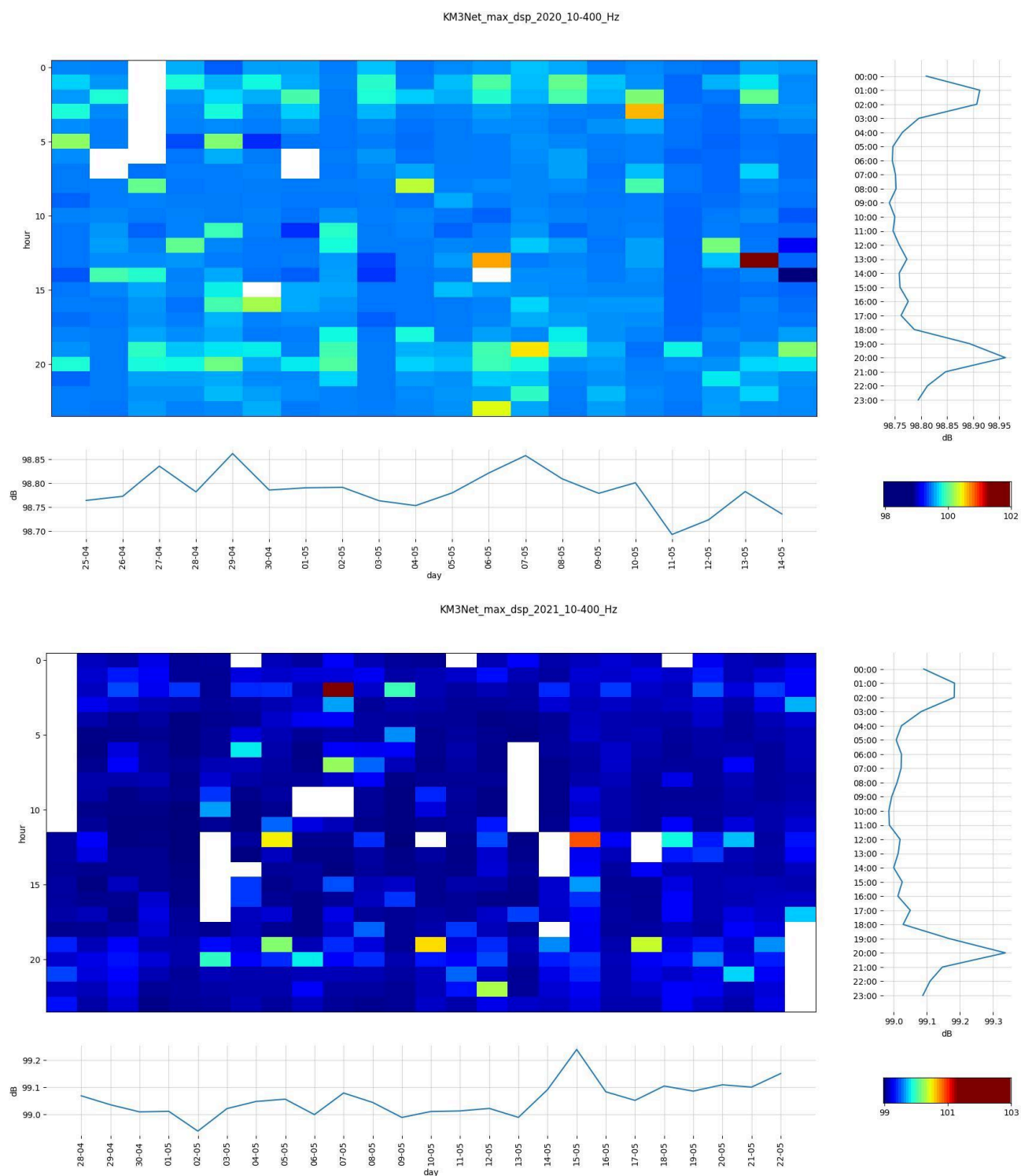
Figure A9.1 : idem, niveau dB maximum par jour sur la bande de fréquence 10 Hz à 800 Hz sur la station KM3Env en 2020 (Haut) et 2021 (Bas) en UTC. Les niveaux maximums sont centrés comme déjà montrés sur 3h à 4h et 21h à 22h (ferries), plus quelques passages de bateaux (carreaux de haute intensité).
