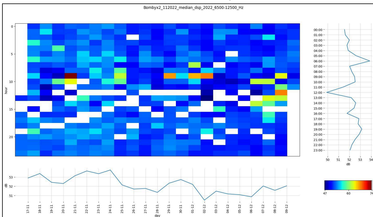
Figure 18.5 : Niveau de bruit médian sur la bande 6.3 kHz à 12.5 kHz de l'hiver 2022 (11 nov. au 7 dec.) montrant un niveau faible de l'ordre de 55 dB la nuit et des passages aléatoires anthropophoniques de +10 à +20 dB.
