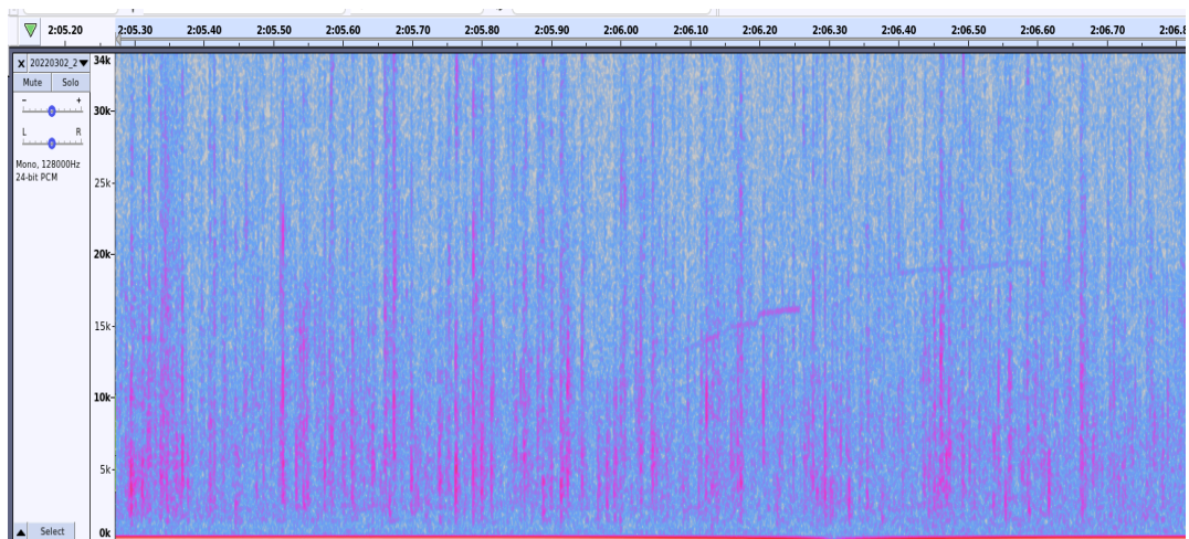
Figure 12.5 : Vocalise d'un odontocète sur Rayol, le 02 mars 2022 à 23h09.
