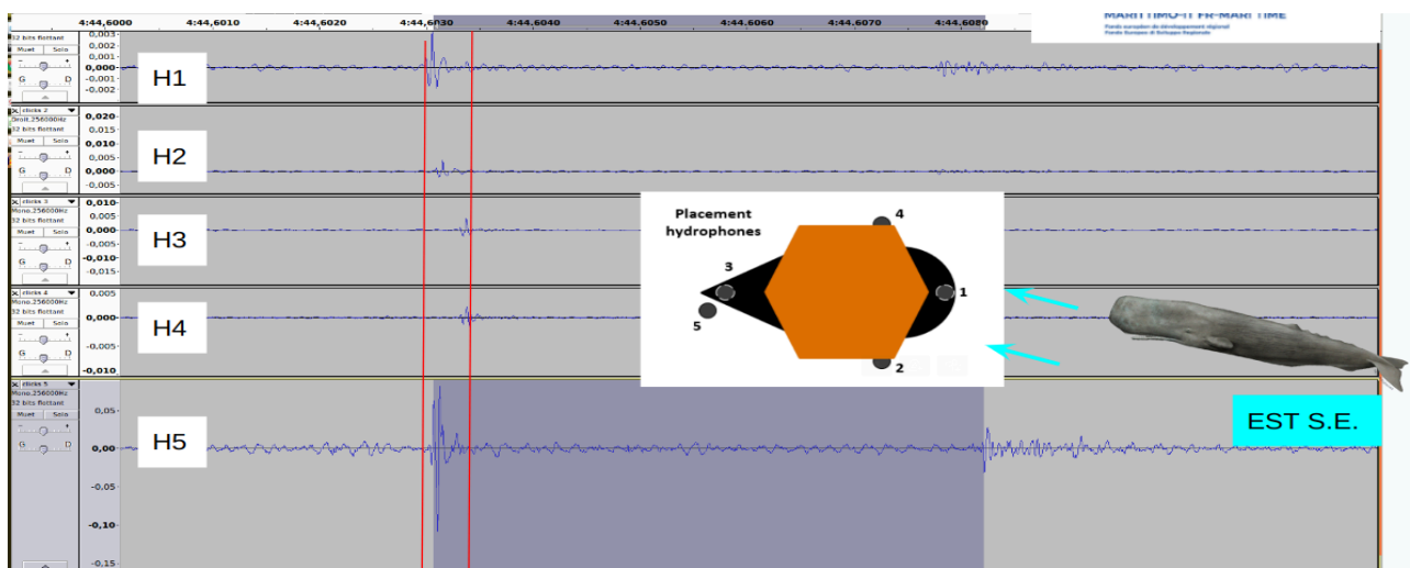
Figure 6.1 : Illustration des mesures de délais d'arrivée des clics d'un cachalot sur BOMBYX-2, sur des hydrophones 1 à 5 rappelés sur le schéma au centre. Ce cachalot est donc placé au SE car la bouée est placée d'Ouest en Est comme figuré, calée dans le courant Ligure, et comme l'indiquent ses mesures de sa Motion Process Unit. On rappelle que H5 est centré, 1.8 m plus bas.
