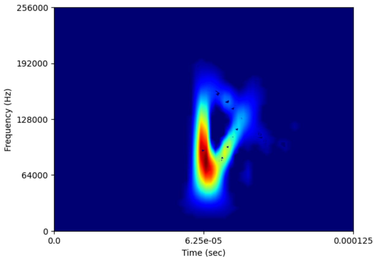
Figure 23.2: Exemple de clics de globicéphale vu au large de Marseille en 2023. Les clics sont représentés par la distribution de pseudo Wigner-Ville à l'échelle du dixième de milliseconde afin d'observer précisément les micros variations spectrales du signal émis.
