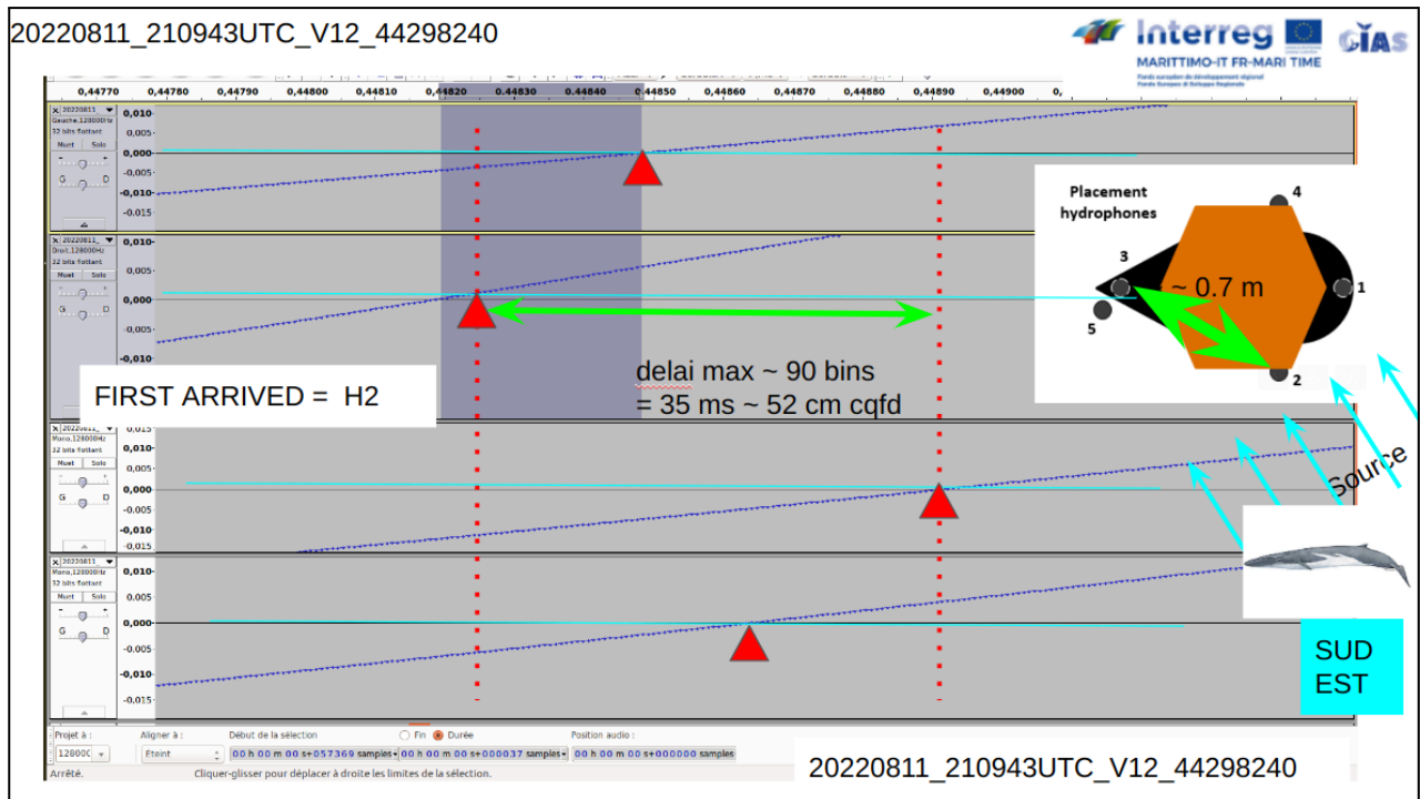
Figure 6.2 : Représentation des arrivées en passage en 0 du pulse de rorqual commun pour estimer les angles d'arrivée, azimuth et élévation du rorqual commun. On rappelle que H5 est centré, 1.8 m plus bas.
