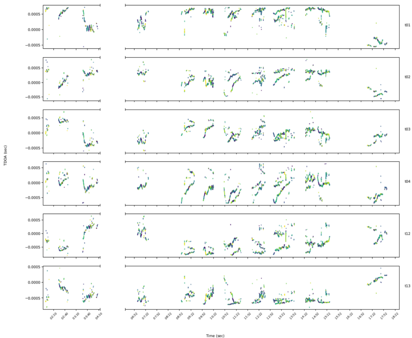
Figure 9.5 : Tracks TDoA de Farouche, Patte d'ours et Casnada durant la journée du 2 octobre 2023, entre 01h48 et 18h01, par JASON Baguera montrant les sondes conjointes.
