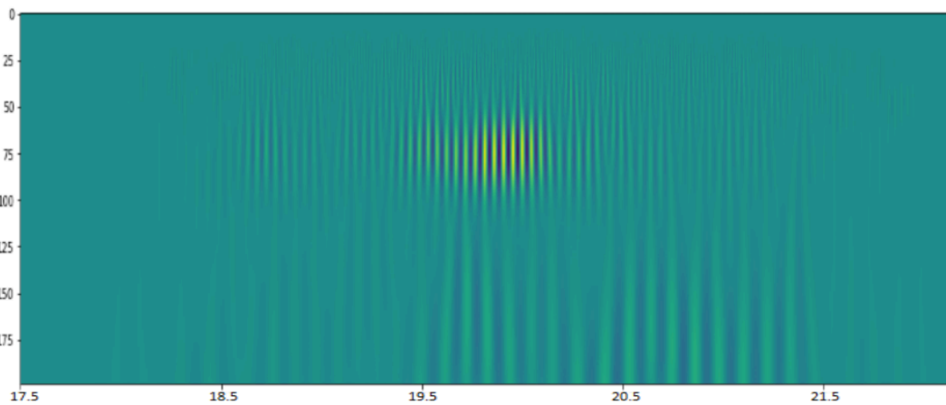
Figure 5.4 : Exemple de décomposition en ondelette de pulse de roqual commun, enregistré en été 2022 par BOMBYX-2 (temps, fréquence).
