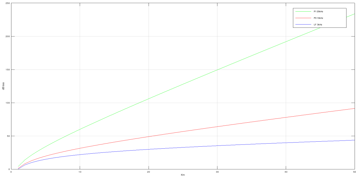
Figure 6.5 : Perte de transmission (dB) des clics 3 kHz (bleu), 10 kHz (rouge) et 20 kHz (vert).
