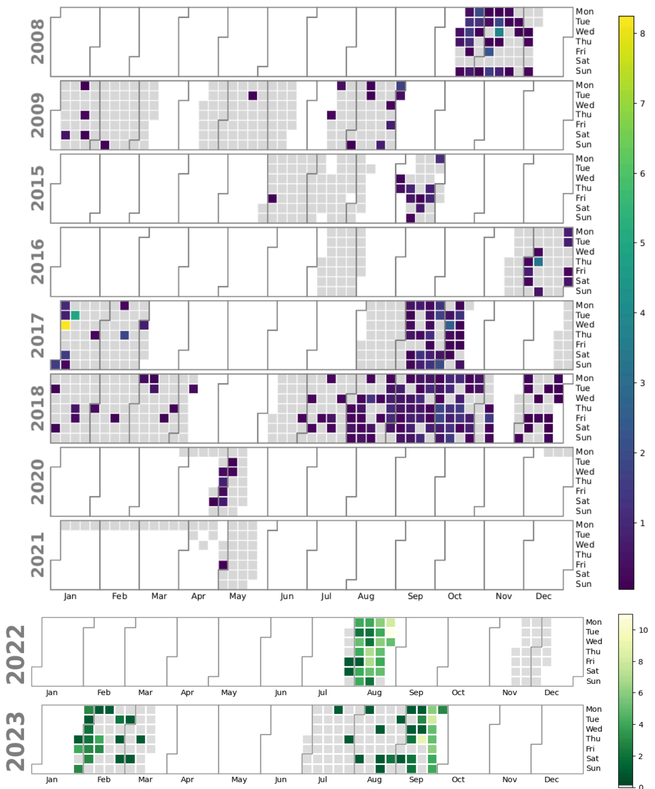
Figure 13.2 : Nombre de trains de pulses de roquhal commun détectés normalisé par le nombre d'heures d'écoute sur Boussole en 2008-2009 (Laran et Glotin et al 2011) et BOMBYX-1 de 2015 à 2018 (Best et al 2022) et KM3Env de 2020 à 2021, et BOMBYX-2 de 2022 à 2023. Les cases blanches correspondent aux jours sans enregistrement, les cases grises aux jours sans détection (seuil de détection positive= 0.75 pour 2022, =0.45 pour 2023, échantillons de 5s).
