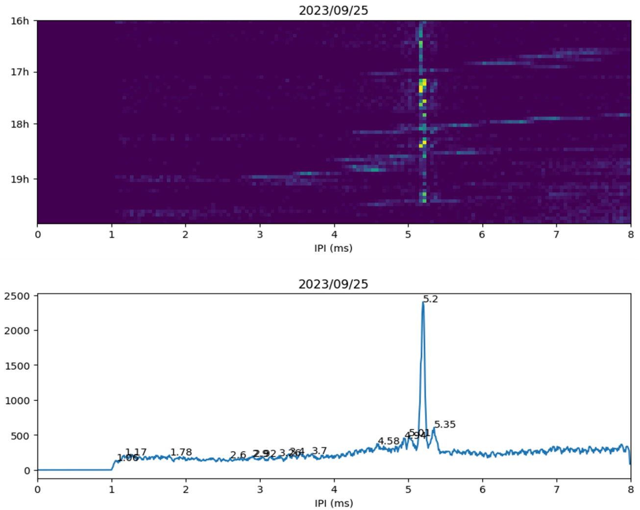
Figure : (Haut) Suivi de la piste en Intervalle inter pulse dans les heures locales (Bas) Histogramme des Intervalles inter pulse de la piste montrant le nombre d'individus et leur IPI, ici Survivor.
