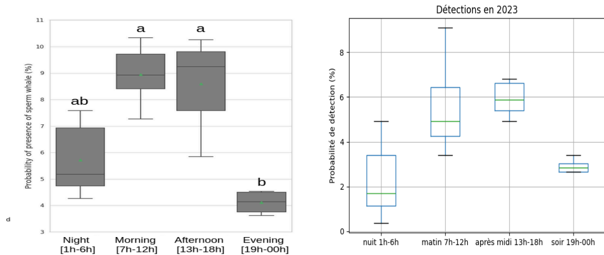
Figure 11.6: (Gauche) Tendance par tranche horaire des détections sur BOMBYX-1 de 2015 à 2018. (Droite) Idem sur BOMBYX-2 en 2023.
