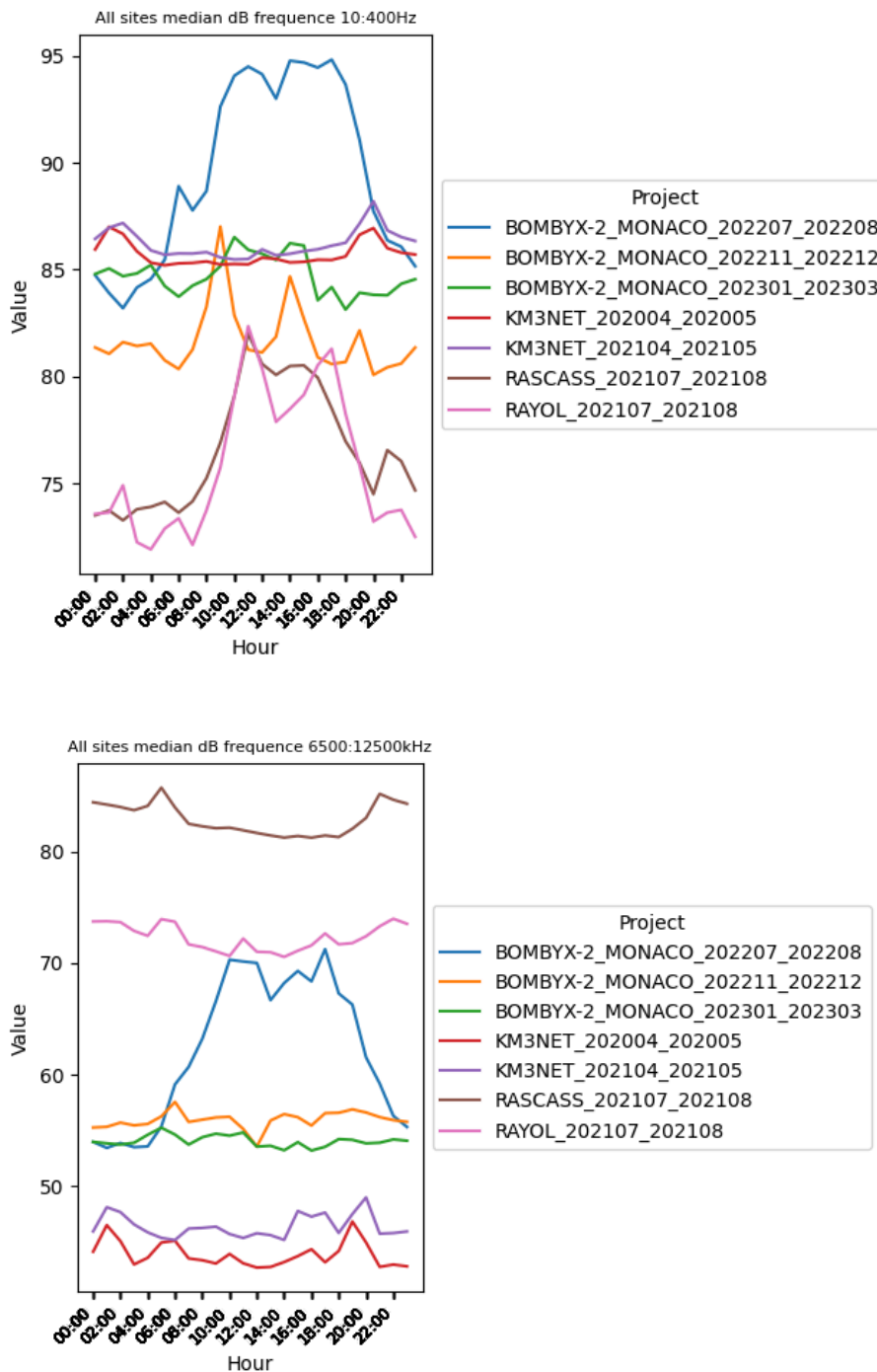
Figure 18.7 : Niveau dB median par heure sur plusieurs mois d'enregistrements des différentes stations pour la bande de fréquence 10-400Hz (haut) et 6500-12500kHz (bas).
