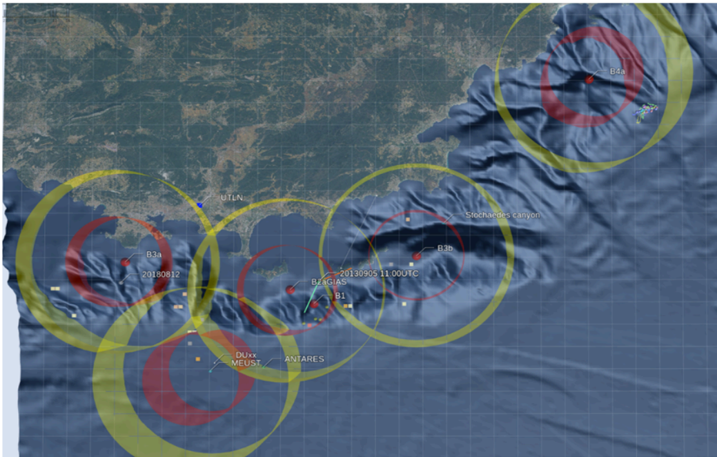
Figure 21.2 : Illustrations en carte dynamique 3D des détections depuis les détections DECAV 2011 ( http://sabiiod.lis-lab.fr/gias/ ) de l'observatoire idéal du projet. Le rayon de détection à haut RSB est de 10 km et à moyen RSB de 20 km (rouge et jaune).
