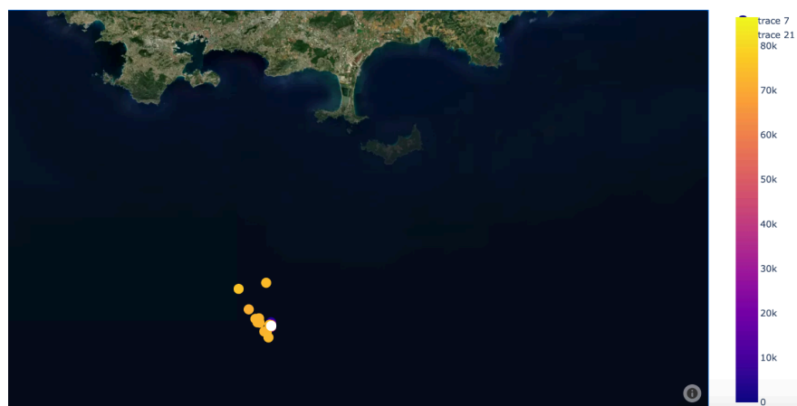
Figure 15.1 : Situation générale de la station KM3Env (point blanc), câblée en fibre optique vers Toulon, avec points de trajectoire d'un rorqual commun, le temps s'écoulant en couleur du bleu 0h00 vers le jaune 23h59 (color bar), pour le 1er mai 2020 (crédit P. Best).
