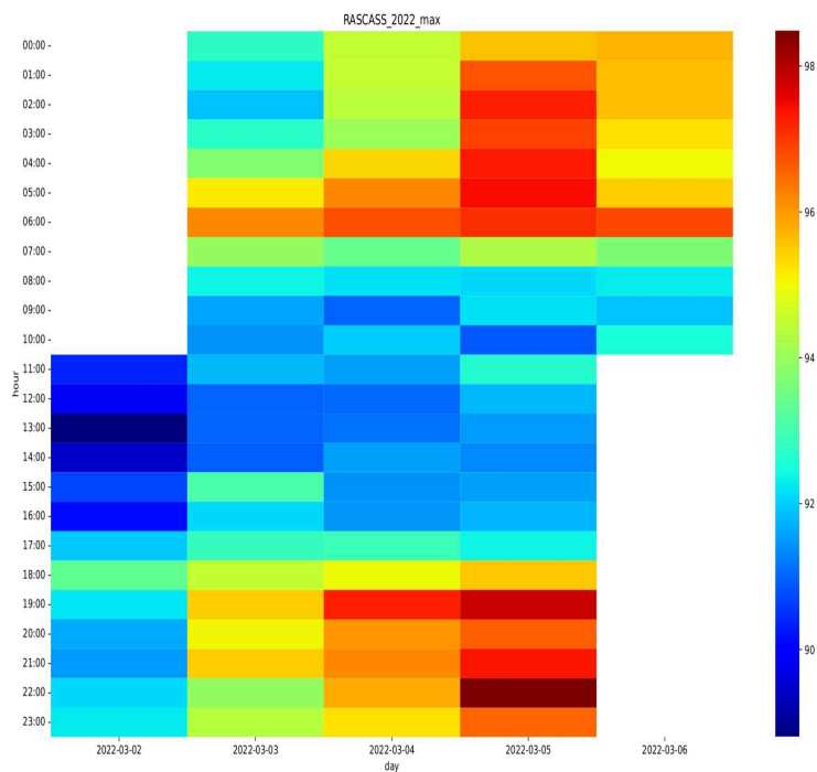
Figure A10.2: Niveau de bruit sur la bande 6300 Hz à 12500 Hz.
