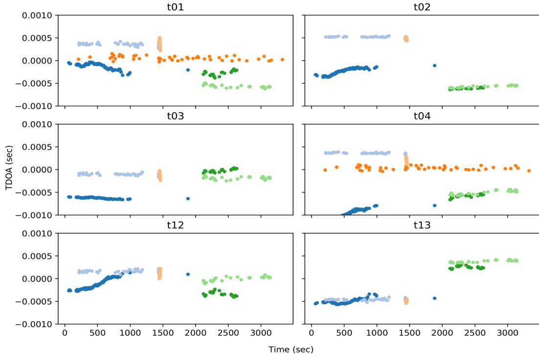
Figure 9.4 : Track TDoA des cachalots Farouche (bleu, rouge et vert foncés) et Patte d'Ours (bleu, rouge et vert clairs) enregistrés le 29 septembre 2023 lors de la sonde de 13h13 à 14h22. Ces tracks montrent qu'ils évoluent suivant les mêmes trajectoires.
