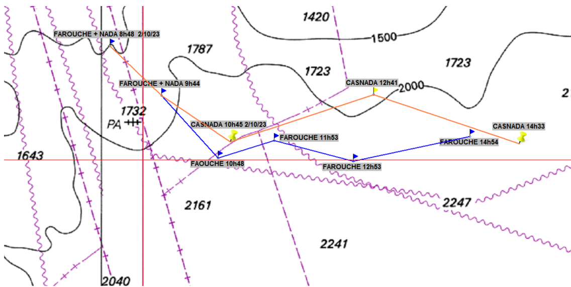
Figure A4.7: (Haut) Suivi réalisé le 02 octobre 2023 pendant la mission WhaleWay. (Bas) Zoom sur le suivi de deux individus.
