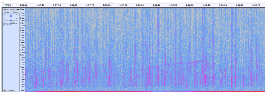
Figure 12.6 : Vocalise d'odontocètes sur Rayol, le 02 mars 2022 à 23h15.
