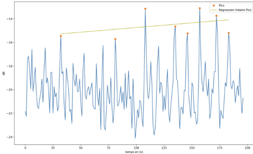
Figure 14.2 : Déplacement non rectiligne d'un rorqual commun sur 3 minutes, avec ses 8 pulses, enregistré le 23 août 2022 sur BOMBYX-2, Monaco (crédit H. Glotin).
