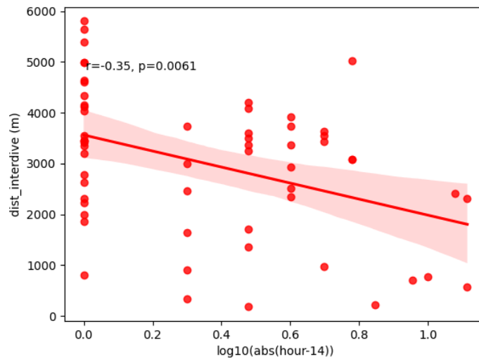
Figure 11.4 : Relation entre l'écart à l'heure solaire et la distance parcourue lors d'une sonde.
