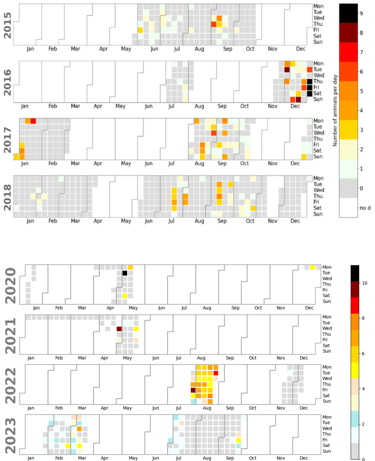
Figure 8.1 : (Haut) Nombre de cachalots détectés par jour sur les 4 années d'enregistrements (zone blanche: pas d'enregistrement) (Poupard et al 2022). (Bas) Calendrier des détections acoustiques : nombre d'enregistrements de 2 min (2020-2021 sur KM3Env) et 5 min (2022-2023 sur BOMBYX-2) ayant au moins trois détections positives de cachalot. Les cases blanches sont les jours sans enregistrement, les grises avec enregistrement mais sans détection. Seuil de détection positive fixé à 0.5, sauf en 2022 fixé à 0.9.
