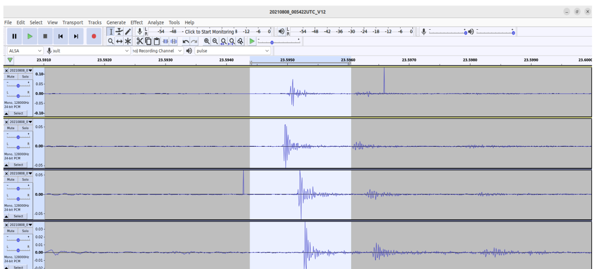
Figure 12.8 : Zoom sur un clic et ses rebonds surface ou fond.
