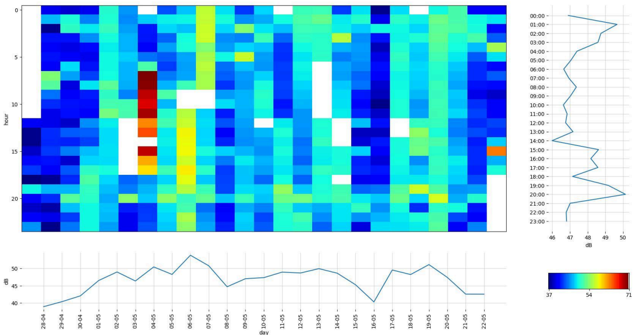
Figure A9.2 : Niveaux dB maximum par jour et heure UTC sur la bande de fréquence 6300 Hz à 12500 Hz sur la station KM3Env en 2020 (Haut) et 2021 (Bas). On note que les perturbations de dB maximum (bandes de 03:00 à 04:00, et de 21:00 à 22:00 locales) sont moins présentes qu'en figure précédente probablement car ces fréquences sont plus directives que les BF de 10 Hz à 400 Hz et donc correspondent à des passages de ferrys plus localisés au-dessus des hydrophones de KM3Env.
