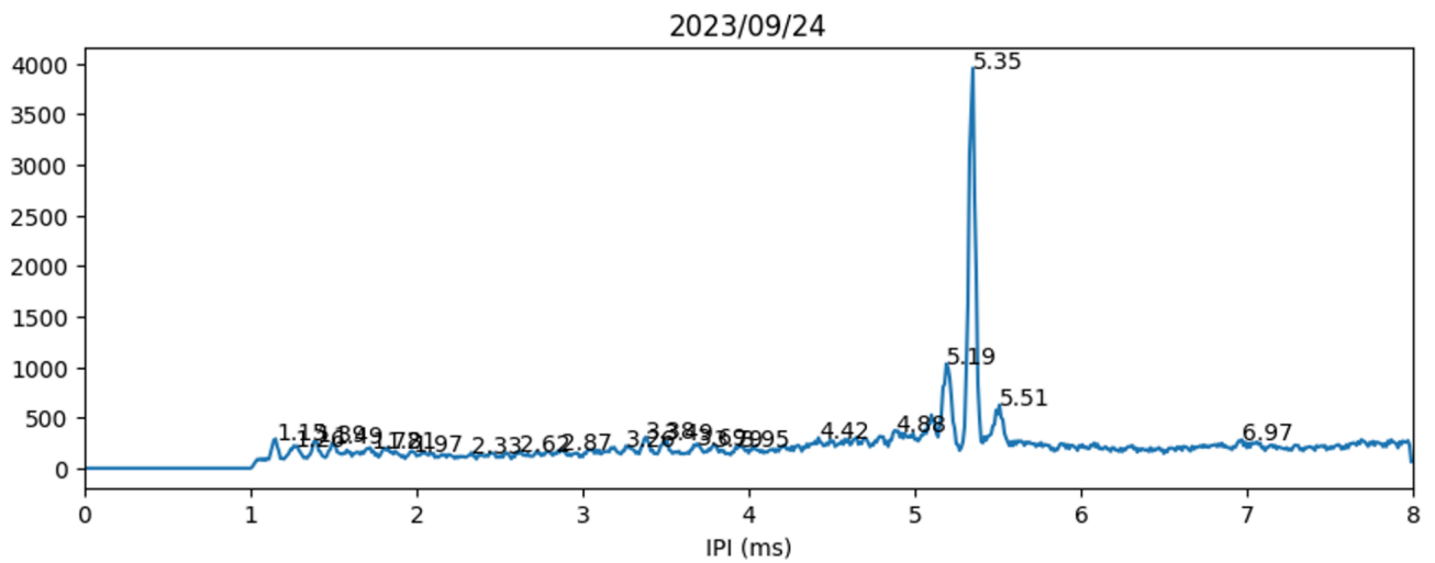
Figure 10.1: (Haut) Suivi de la piste en Intervalle inter pulse dans les heures. (Bas) Histogramme des Intervalles inter pulse de la piste montrant le nombre d'individus et leur IPI. Ici Cyclone, IPI de 5,35 ms.
