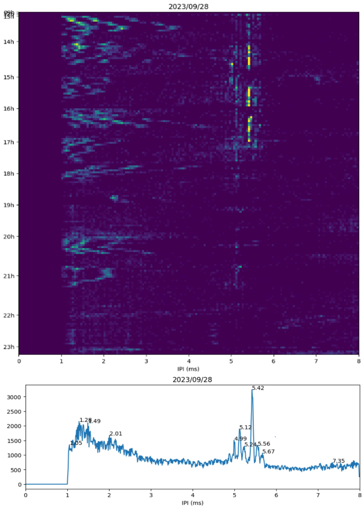
Figure 10.2: (Haut) Suivi de la piste en Intervalle inter pulse dans les heures. (Bas) Histogramme des intervalles inter pulse de la piste montrant le nombre d'individus et leurs IPI, ici Jupiter (5,42ms), ZZtop (5,67ms), Plune (5,56ms) et Farouche (5,12ms).
