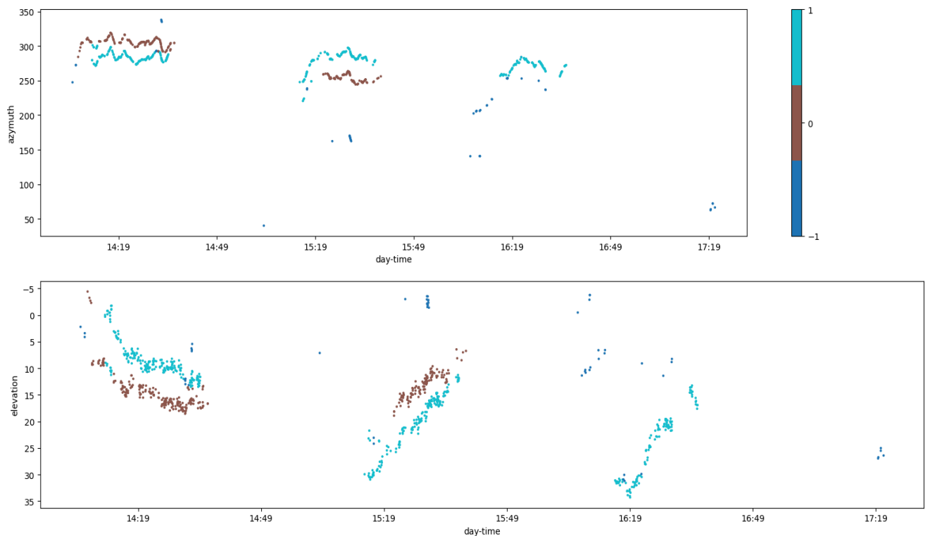
Figure 9.7 : Suivi des mesures d'azimut et d'élévation de Farouche et Nada le 1er octobre de 14:19 à 17:19, donc durant 3h, et plongeant ensemble durant 3 plongées (Fig. 9.8). Ces motifs démontrent la coordination de leurs sondes, même en milieu anthropisé. (marron: Nada IPI 5.05ms, bleu clair : Farouche IPI 5.14). La 3ème sonde ne montre qu'une piste Farouche, mais les deux ont sondé, Farouche est donc silencieux à l'écoute de Nada.
