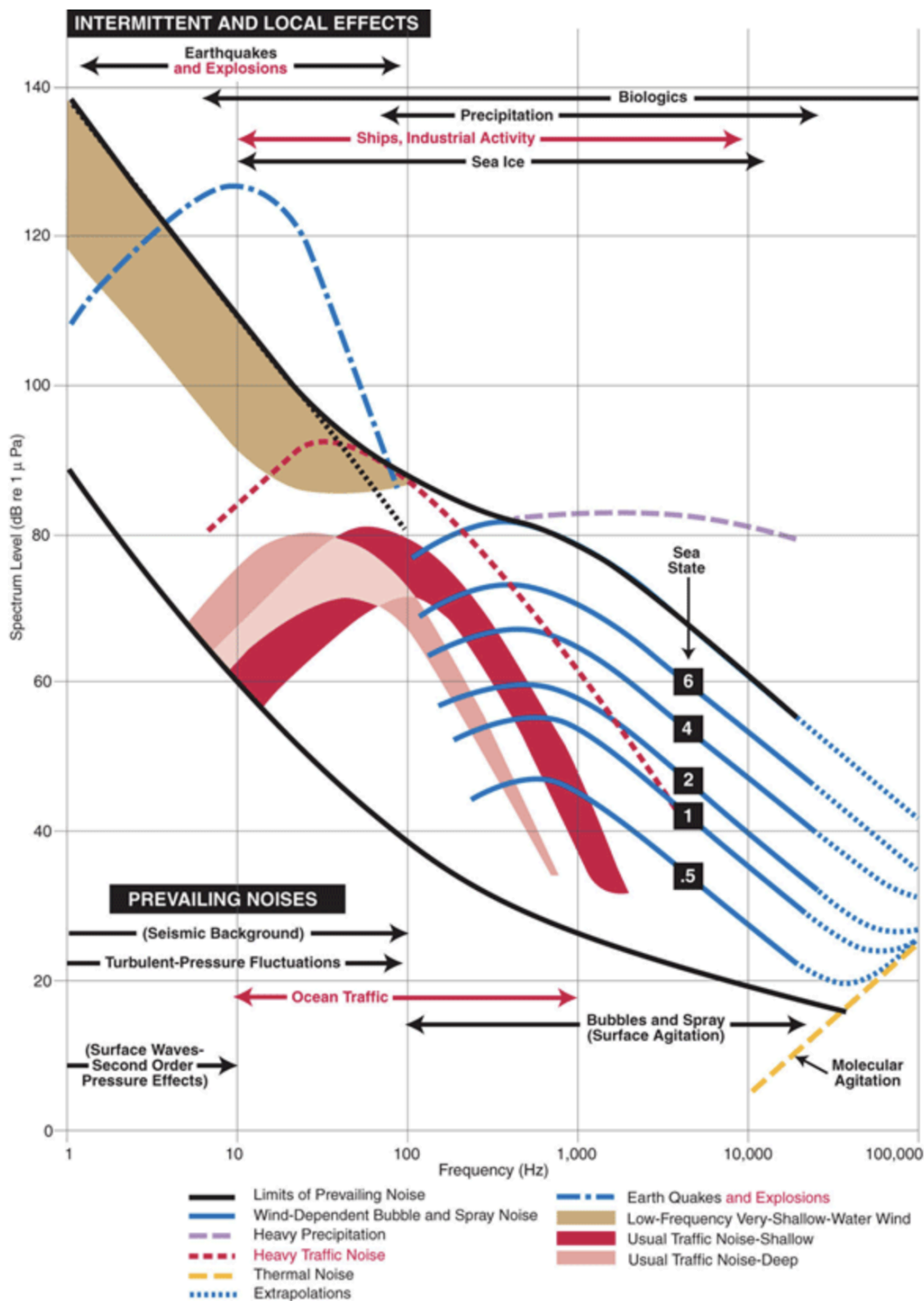
Figure 7.1 : Les niveaux dB de référence (d'après Wenz 1962).
