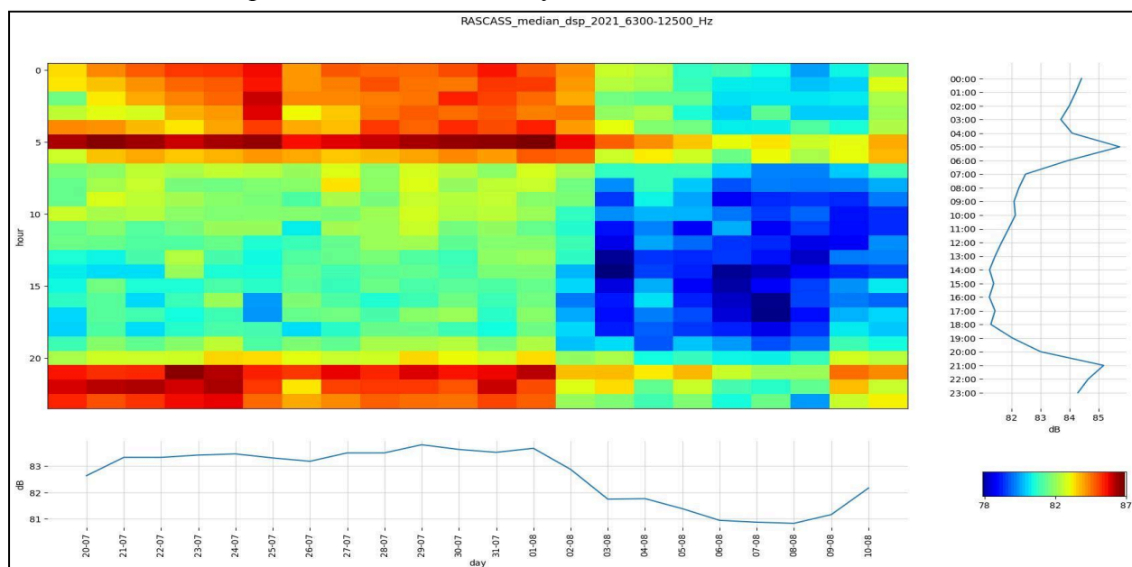
Figure 17.3 : Niveau dB médian sur la bande 6.3 kHz à 12.5 kHz, du 19 juillet au 11 août 2021 pour Rascass. On constate un plateau de bruit de 21h00 à 05h00, probablement lié à l'activité du plancton et des récifs plus actifs la nuit. Toujours pas de bruit de ferry. La chute des bruits le 2 août est corrélée à la température, cf infra.
