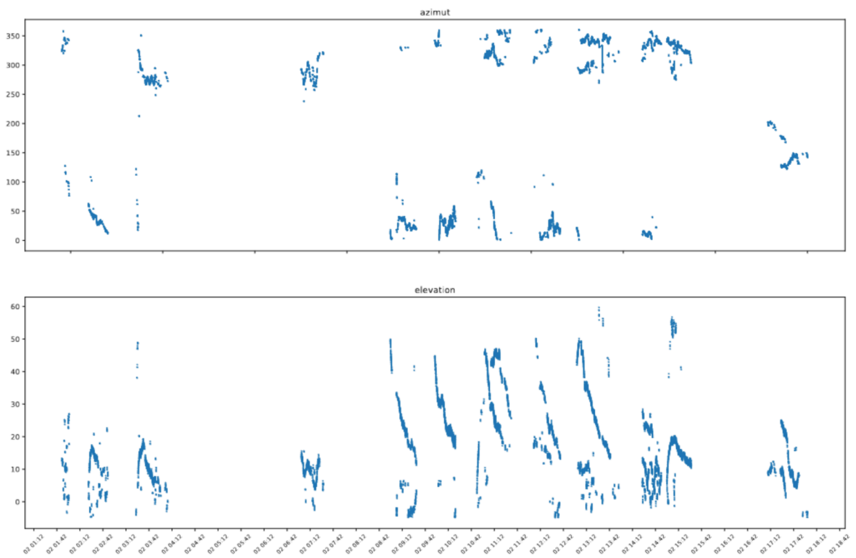
Figure 9.9 : Suivi des mesures d'azimut et d'élévation de trois individus plongeant ensemble : Farouche, Casnada et Inattendu, enregistrés durant la nuit et la journée du 2 octobre 2023, de 1h12 à 18h42.
