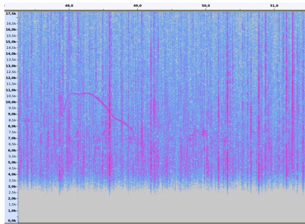
Figure 12.3 : Spectrogramme représentant des sifflements de delphinidés (08/08/2021 à 03h05).
