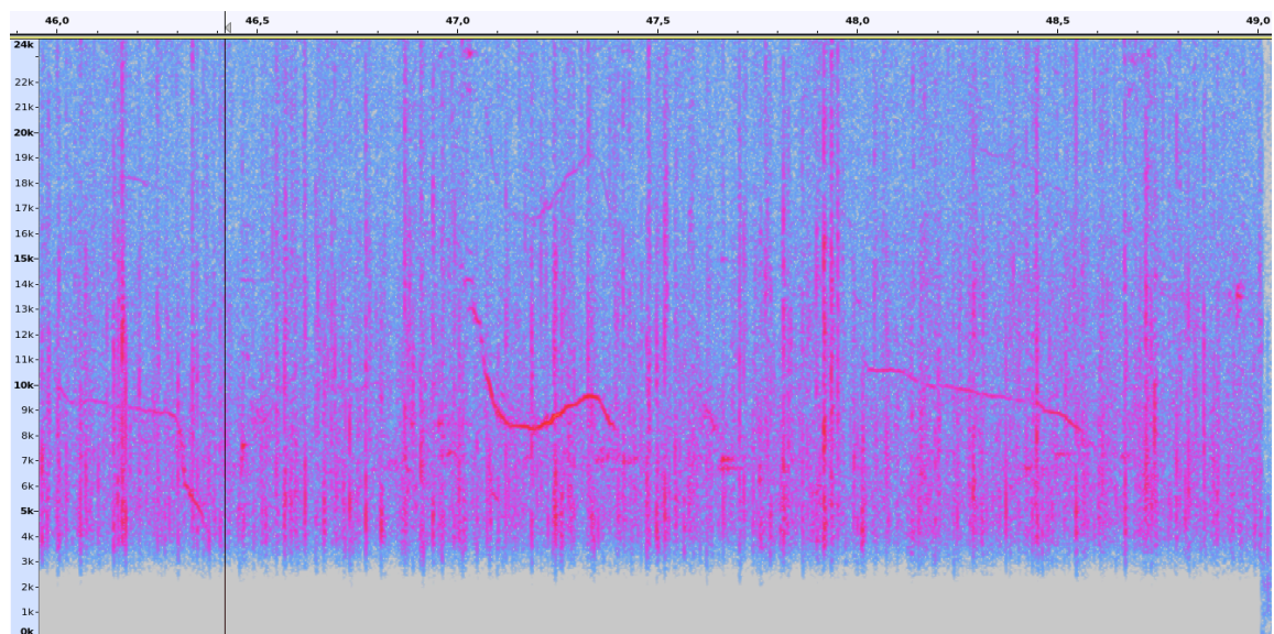
Figure 12.2 : Spectrogramme représentant des sifflements de delphinidés (08/08/2021 à 00h54).
