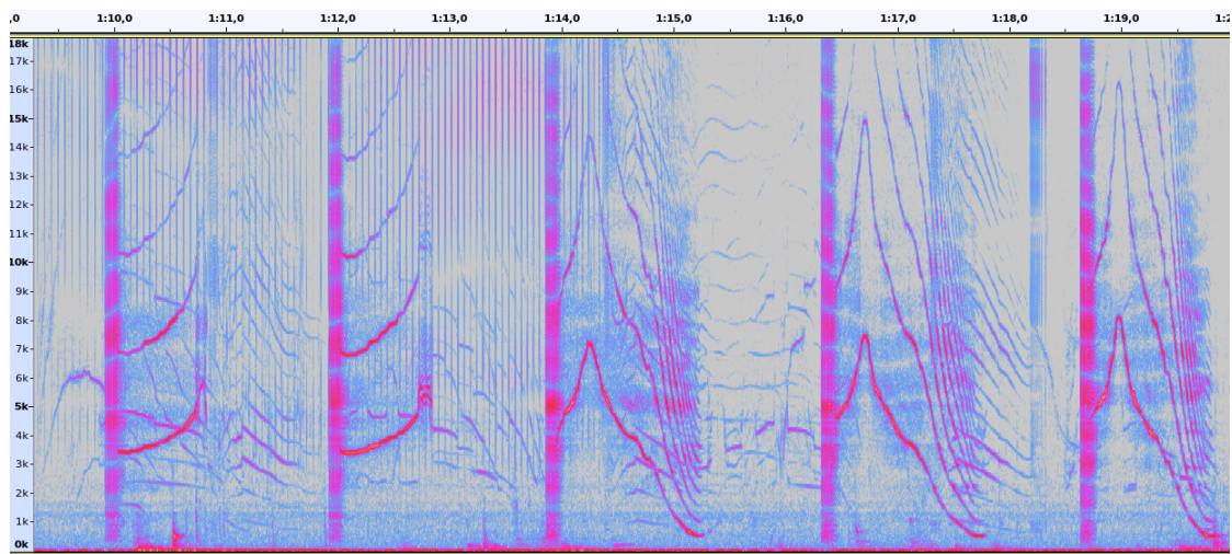
Figure 23.1: Exemple de vocalises de globicéphales vers Marseille en 2020. Le spectre de 20 kHz de largeur est complexe. Ces formes pourraient porter une information clanique qui pourrait être identifiée par IA (cf le premier répertoire de ces formes pour la Méditerranée Poupard et al 2024). Cette approche permettrait de suivre les populations sous pressions anthropiques/ climatiques.
