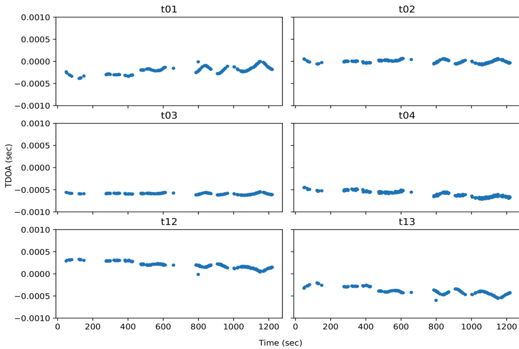
Figure 9.3 : Track TDoA du cachalot ZZ-top enregistré, le 27 septembre 2023 lors de la sonde de 14h, par JASON Baguera. Début de l'enregistrement à 14h43 et fin à 15h04. Les 6 affichages représentent 6 couples d'hydrophones différents tels que t01 est le temps d'arrivée entre l'hydrophone 1 et l'hydrophone 2, t02 entre l'hydrophone 1 et l'hydrophone 3, et ainsi de suite.
