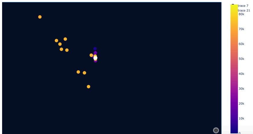
Figure 15.3 : Zoom sur des exemples de trajectoires 2D de rorqual commun calculées sur les trois hydrophones de KM3Env, le 1er mai 2020. KM3Env est le point blanc (crédit P. Best).
