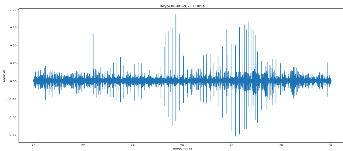
Figure 12.7 : Trains de clics détectés entrelacés de 2 ou 3 dauphins. On mesure un ICI de 0,1 sec environ pour les plus grands ICI.
