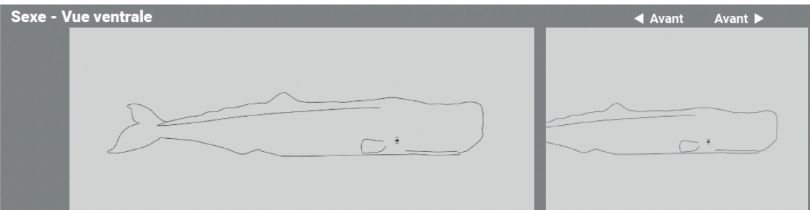
Figure A16.2 : Fiche d'identité du cachalot Farouche qui a été revu 5 jours de suite, chaque fois en compagnie d'un autre individu, lui aussi identifié.
