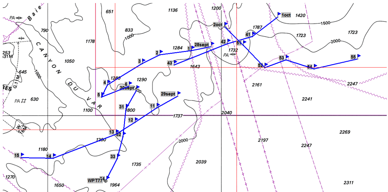
Figure 9.2 : Compilation des trajets d'un unique cachalot, nommé Farouche. Suivi en cumulé sur 5 jours, démontrant l'intérêt de l'habitat Canyon du Var pour cet individu.
