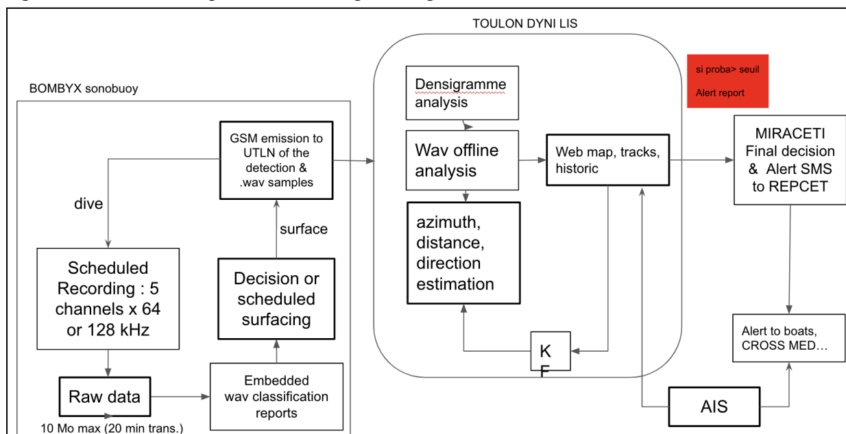
Figure 21.4 : Schéma général du système BOMBYX d'alerte anti-collision.
